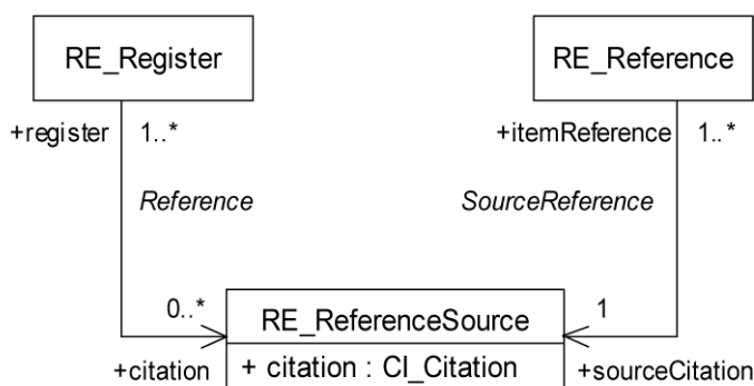
Figure 13 — RE_ReferenceSource
